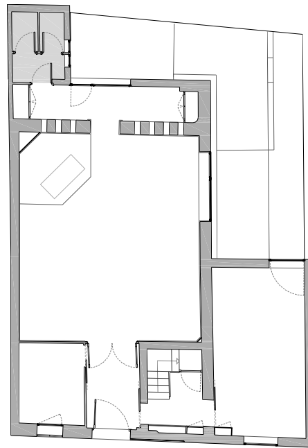
PLANTA BAJA 0 1 2 3 4m
